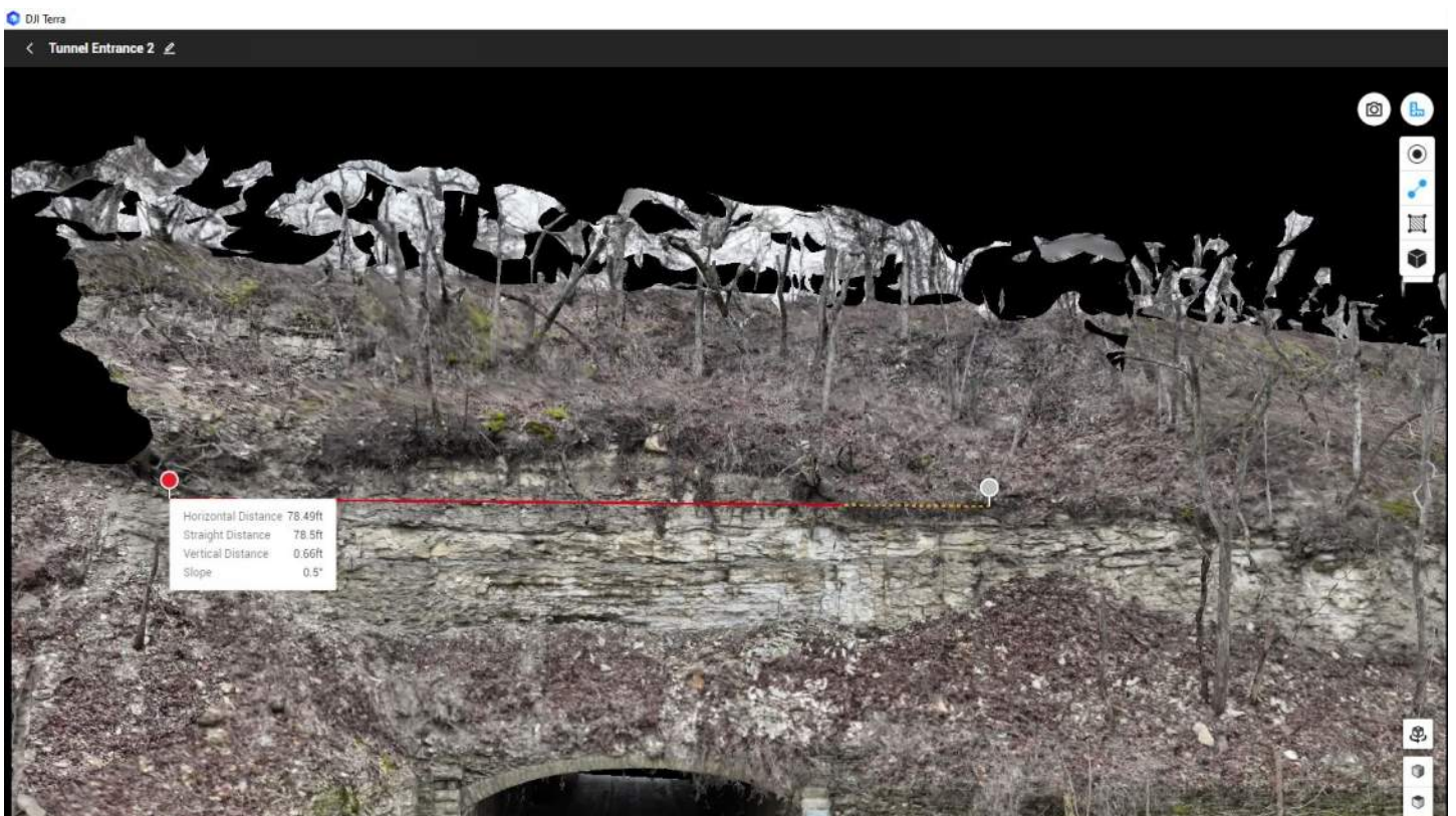
NE Bluff Top Dimension
